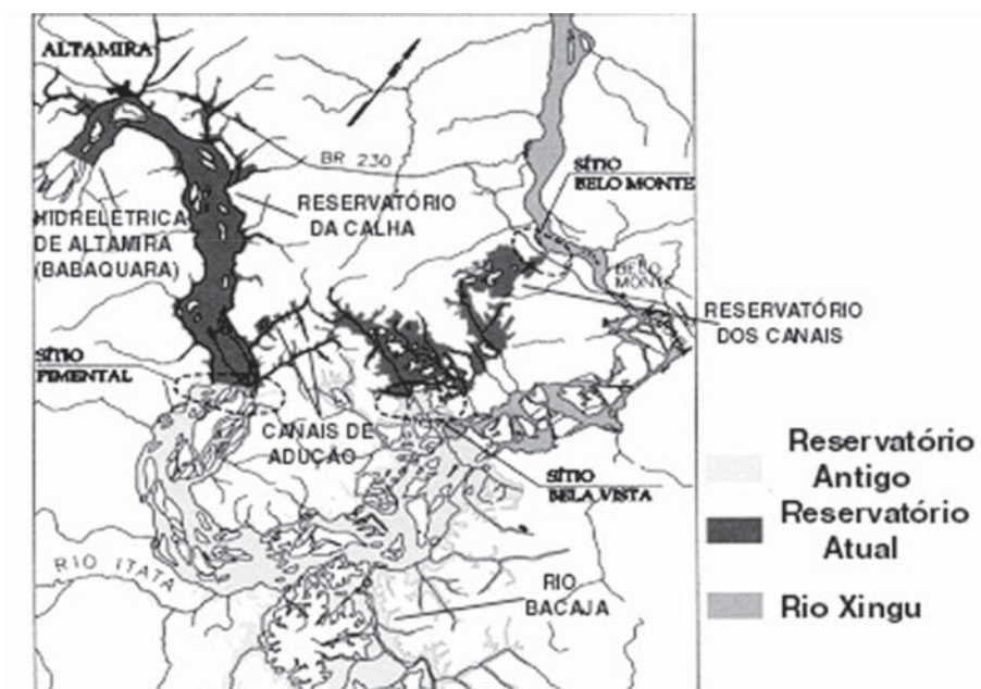
Figura 1. A.) Babaquara (Altamira) Reservatório; B.) Reservatórios de Belo Monte da Calha e dos Canais. Fontes: Babaquara: ELETRONORTE, [1988]; Belo Monte: ELETRONORTE, [2002a].
